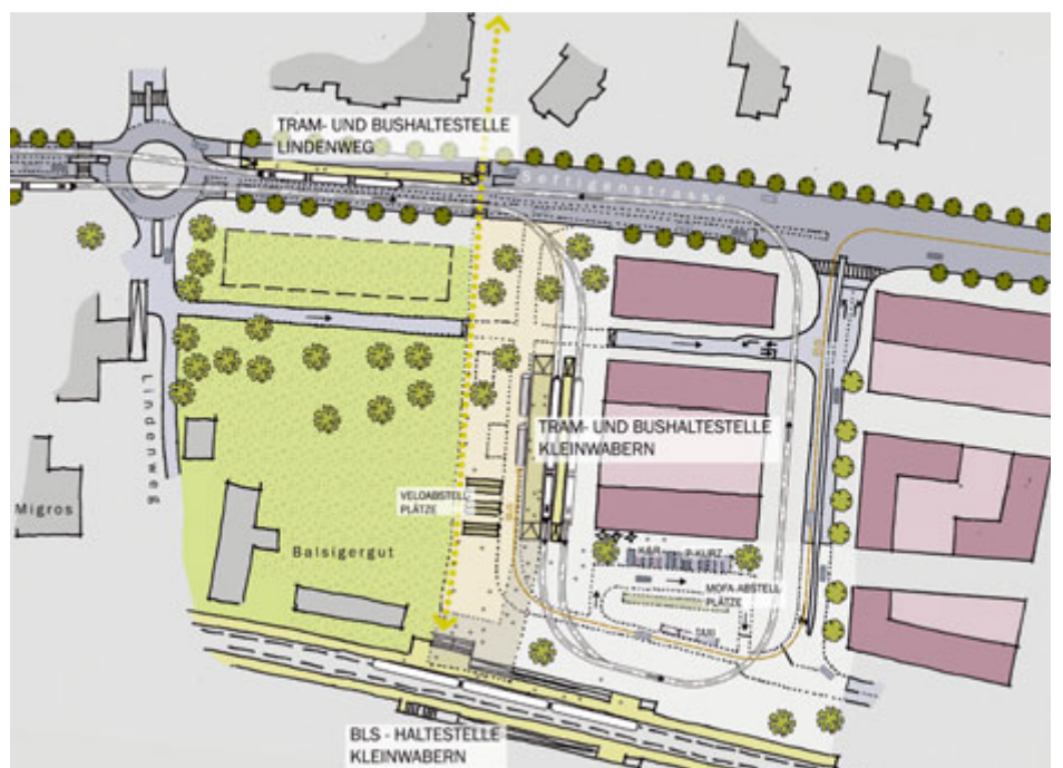
Schematische Darstellung der Situation in Kleinwabern: Die Tramhaltestelle liegt rechtwinklig zur neuen S-Bahnstation und der Seftigenstrasse.
