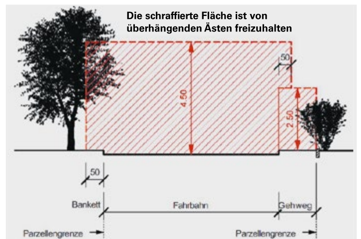
Lichtraumprofil Strasse
